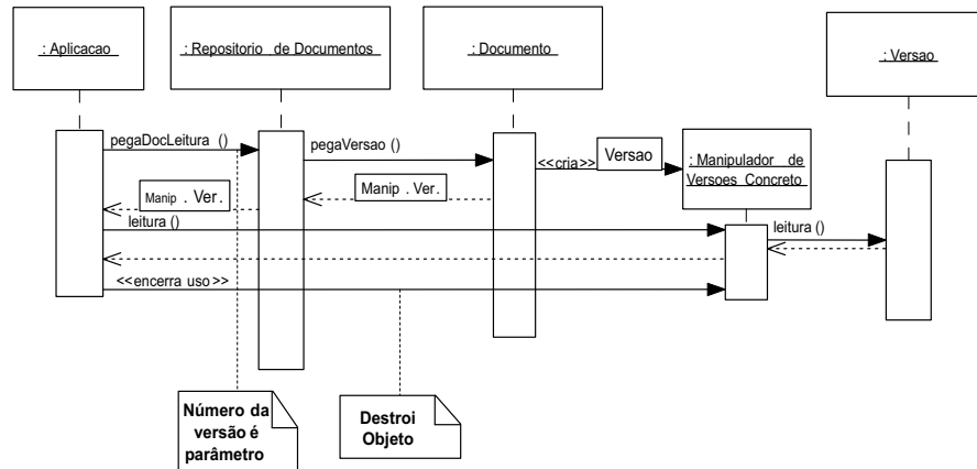
Figura 2: Diagrama de seqüência para leitura de documento.
