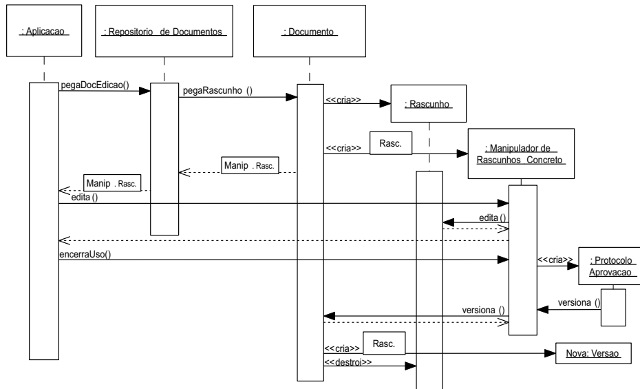
Figura 3: Diagrama de seqüência para edição de documento.
